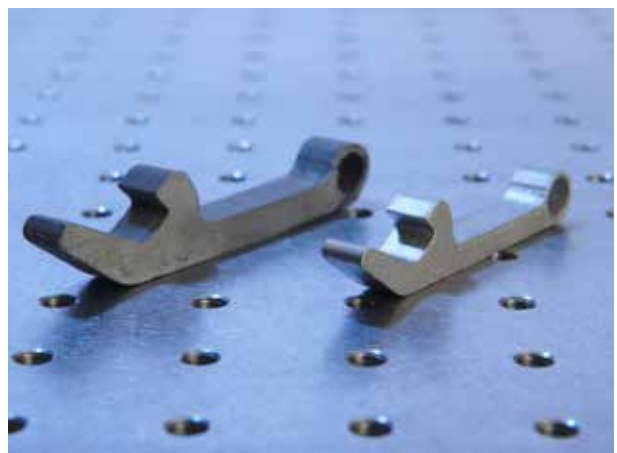
Binder Jetting (links: Grünling, rechts: fertiges Bauteil)
