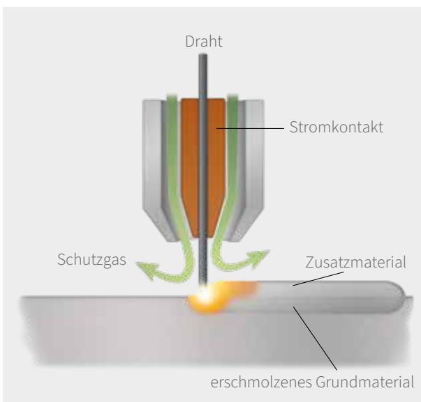
Direct Energy Deposition - Arc (DED-Arc) mit Draht
